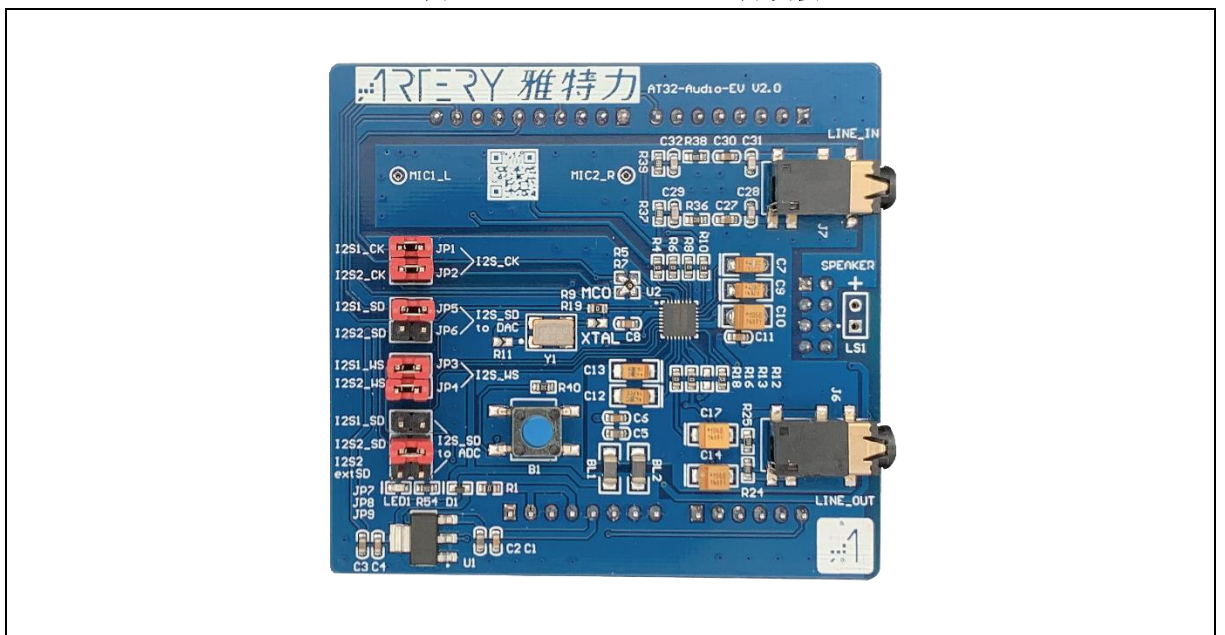
图 2. AT32-Audio-Ev v2.0 开发板
